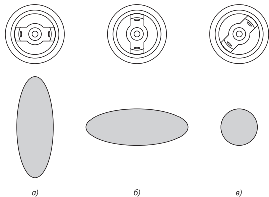
Рис. 2. Форма факела в зависимости от положения форсунки
