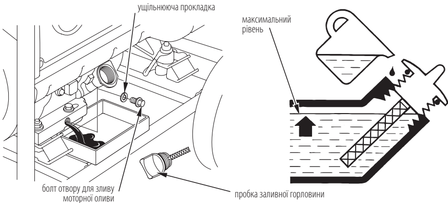
Мал. 8. Заміна оливи
