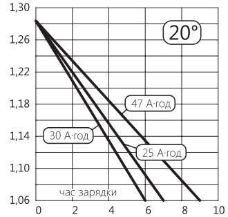
Таблиця 2. Визначення необхідного часу зарядки
